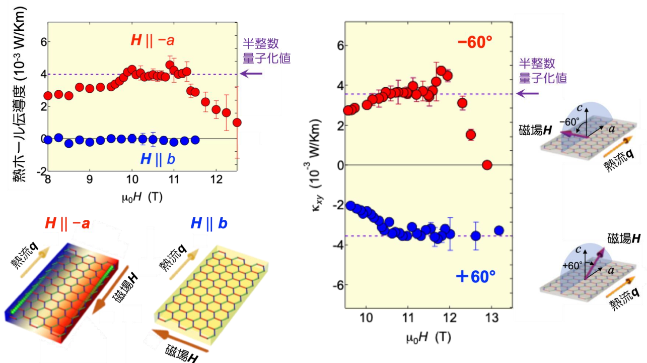
図1：（左上）面内磁場( H \parallel -a , H \parallel b )における \alpha -RuCl 3 の熱ホール伝導度の磁場依存性。 H \parallel -a において、磁場を変化させると、ある磁場範囲で熱ホール伝導度が量子化熱伝導度の1/2で一定となり、半整数熱量子ホール効果が観測された。一方、 H \parallel b では熱ホール伝導度はほぼゼロとなった。（左下） H \parallel -a , H \parallel b における熱ホール効果のイメージ図。（右）傾斜磁場( \pm 60^\circ )における熱ホール伝導度の磁場依存性。 +60^\circ と -60^\circ で半整数熱量子ホール効果の符号が反転する。
